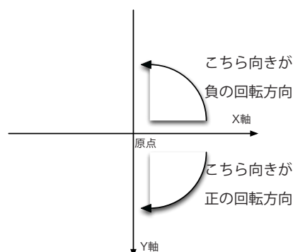
図 6-7 回転の向き
