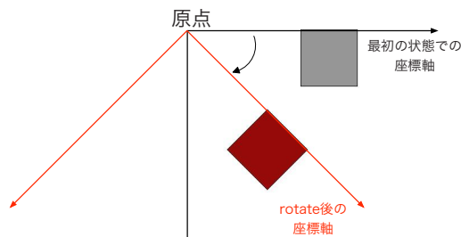
図 6-8 rotate 前後の座標軸
